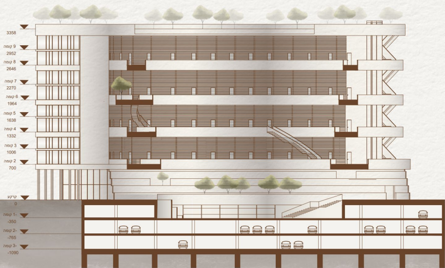
חתך א-א | 1:200
