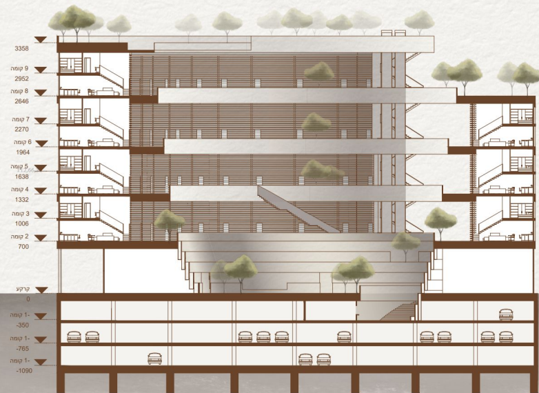
חתך ב-ב | 1:200
